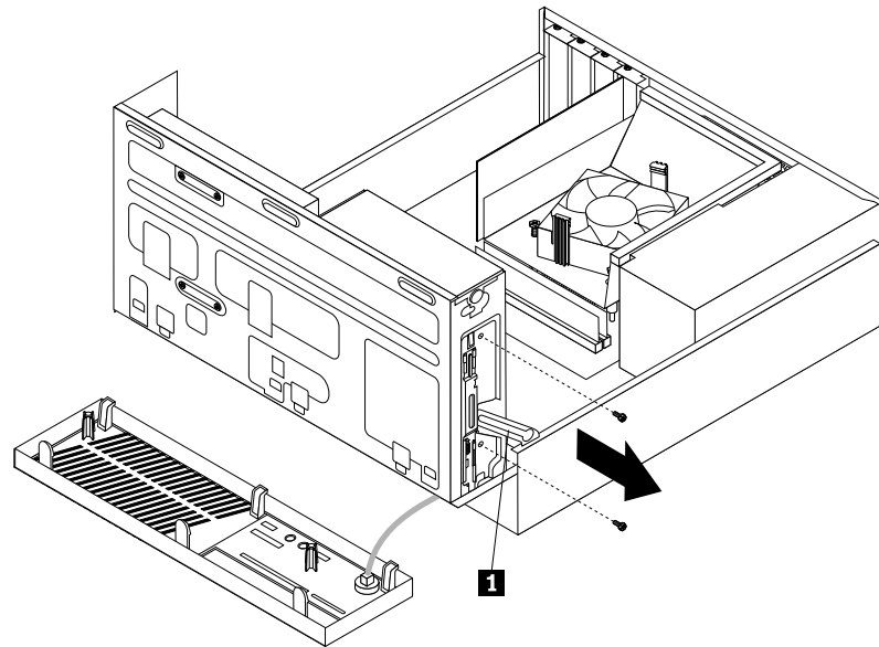
Abbildung 32. Schrauben des optischen Laufwerks entfernen
