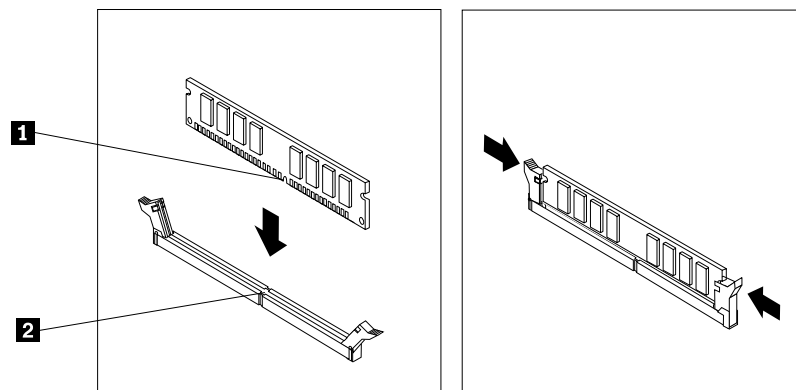
Abbildung 16. Speichermodul installieren
