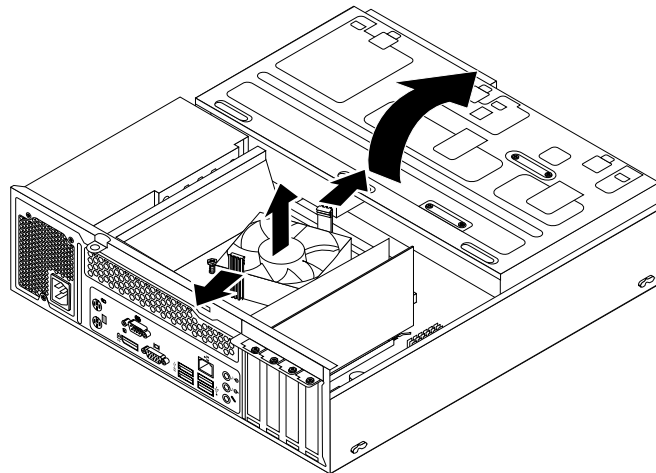
Abbildung 38. Kühlkörperlüftungskanal entfernen
