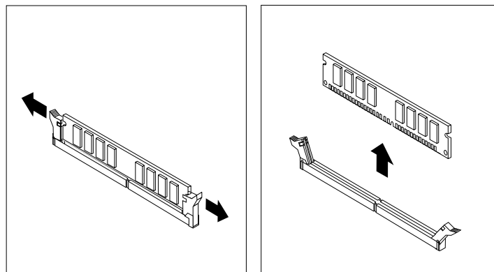
Abbildung 14. Speichermodul entfernen
