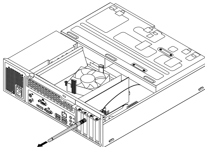
Abbildung 60. Hintere WiFi-Antenne entfernen
