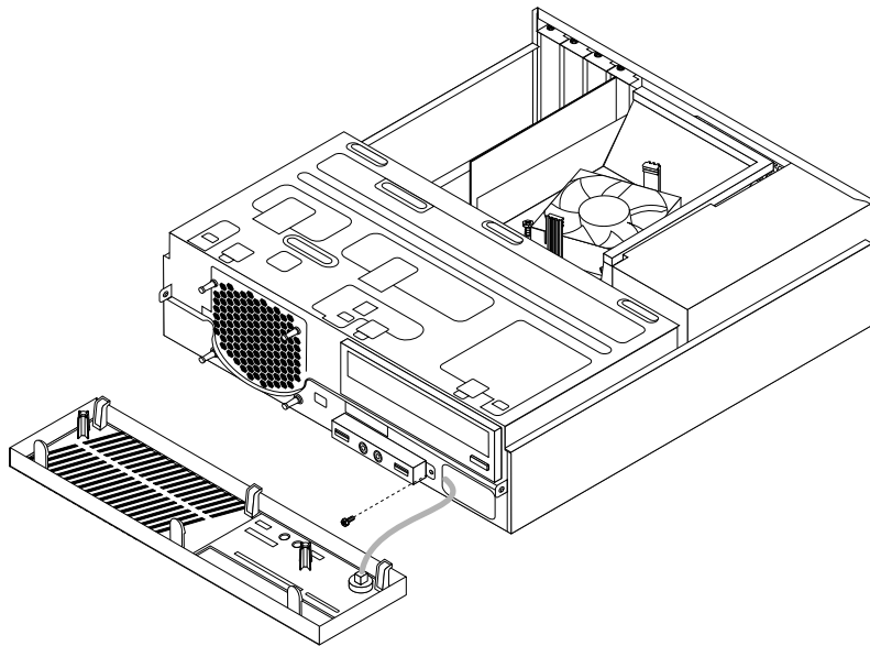
Abbildung 48. Audio- und USB-Baugruppe an der Vorderseite entfernen
