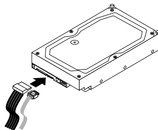
Abbildung 23. SATA-Festplattenlaufwerk anschließen
