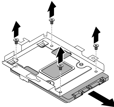
Abbildung 28. Solid-State-Laufwerk aus der Halterung entfernen
