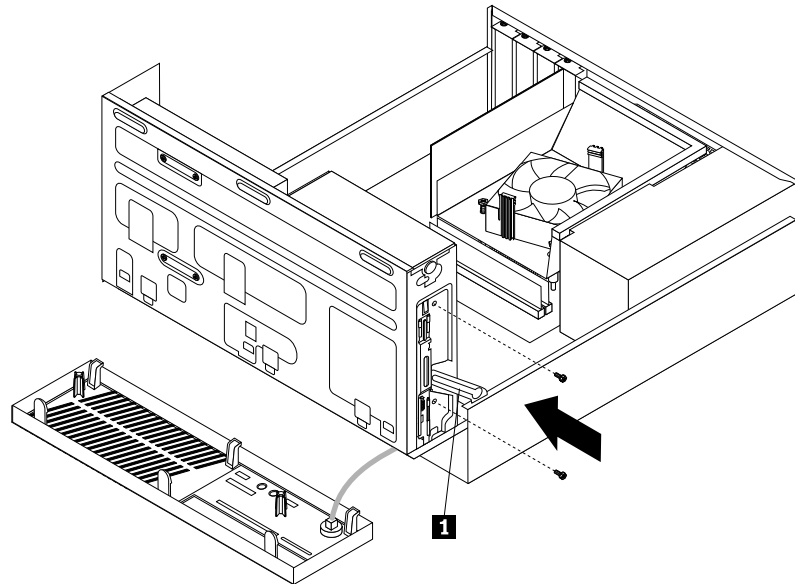
Abbildung 36. Optisches Laufwerk installieren
