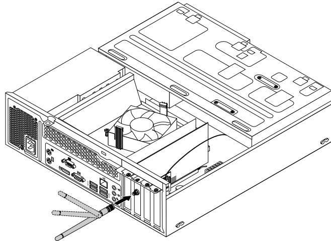
Abbildung 59. Hintere WiFi-Antenne anbringen
