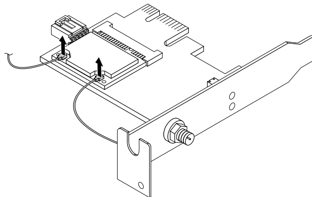
Abbildung 53. WiFi-Antennenkabel entfernen
