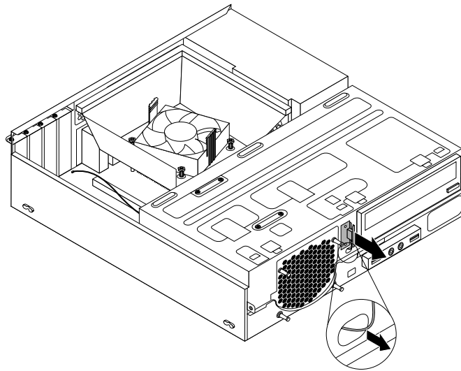
Abbildung 63. Vordere WiFi-Antenne entfernen
