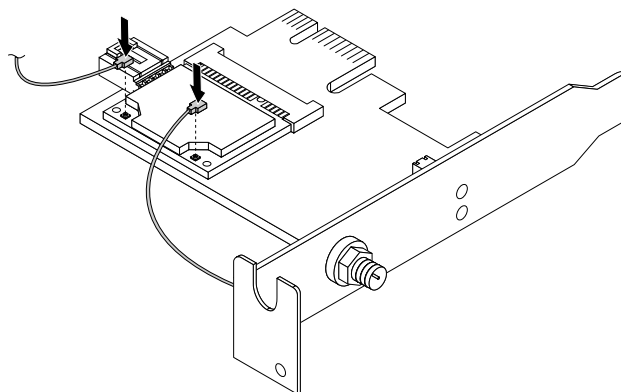
Abbildung 57. WiFi-Antennenkabel anschließen
