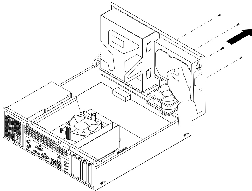
Abbildung 22. Festplattenlaufwerk entfernen
