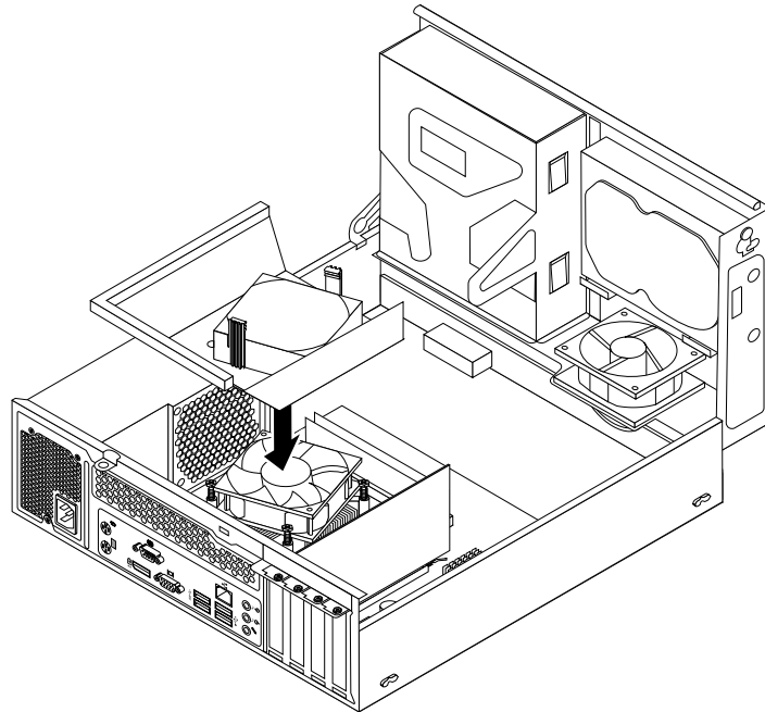
Abbildung 44. Kühlkörperlüftungskanal installieren
