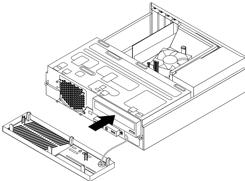
Abbildung 35. Neues optisches Laufwerk installieren
