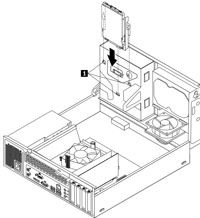
Abbildung 30. Halterung des Solid-State-Laufwerks einbauen
