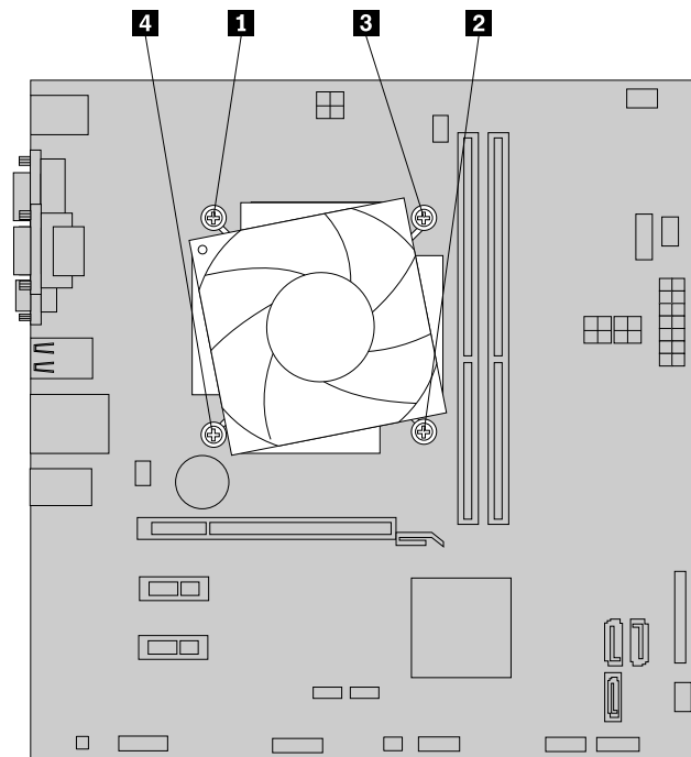
Abbildung 39. Kühlkörper- und Lüftungsbaugruppe entfernen
