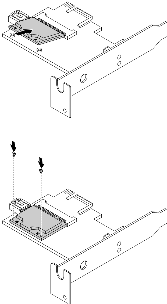
Abbildung 56. WiFi-Kartenmodul installieren
