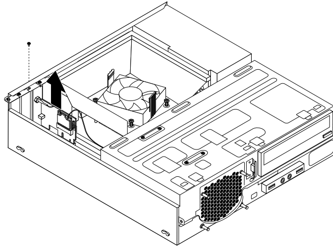
Abbildung 52. WiFi-Adapterkarte entfernen
