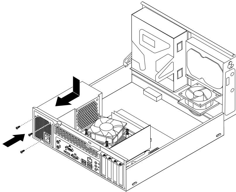
Abbildung 43. Netzteil installieren
