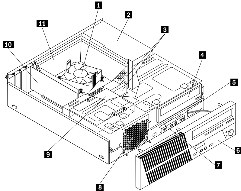
Abbildung 3. Positionen der Komponenten
