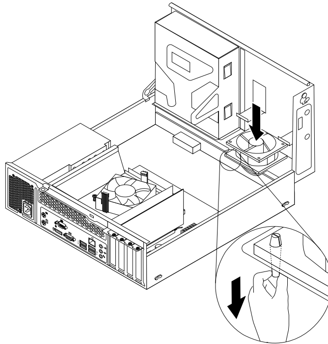
Abbildung 50. Systemlüftungsbaugruppe installieren
