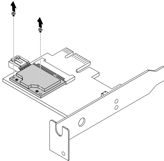
Abbildung 54. Die Schrauben, mit denen der WiFi-Kartenmodul befestigt ist, entfernen
