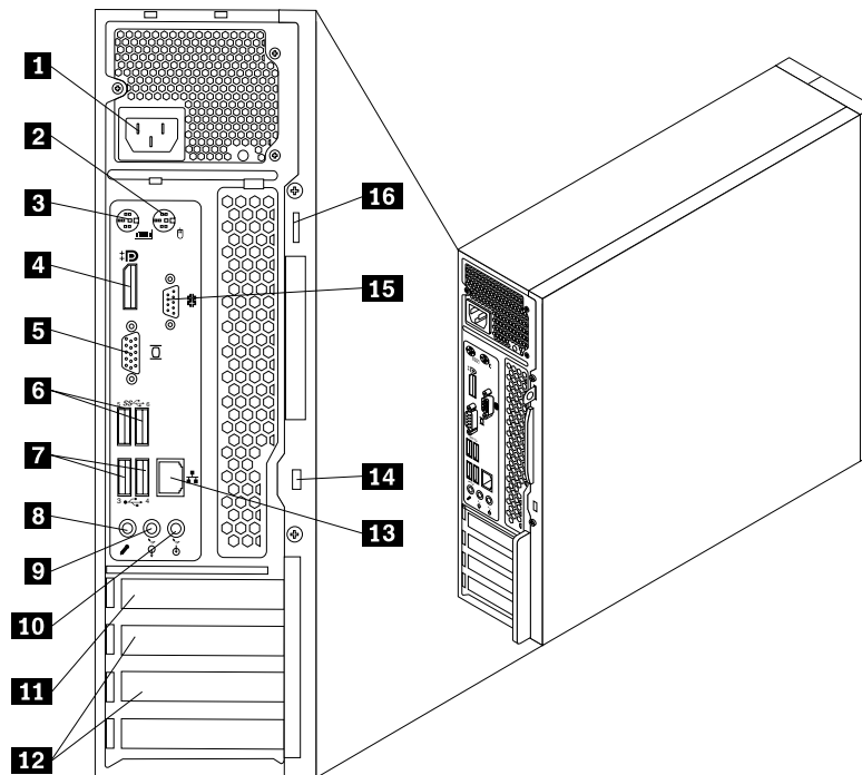
Abbildung 2. Positionen der Anschlüsse an der Rückseite
