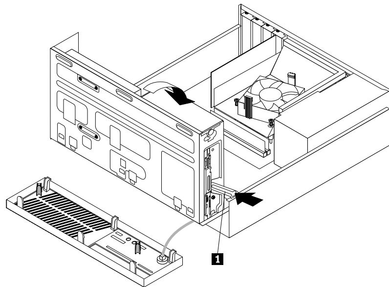
Abbildung 13. Absenken der Laufwerkpositionsbaugruppe
