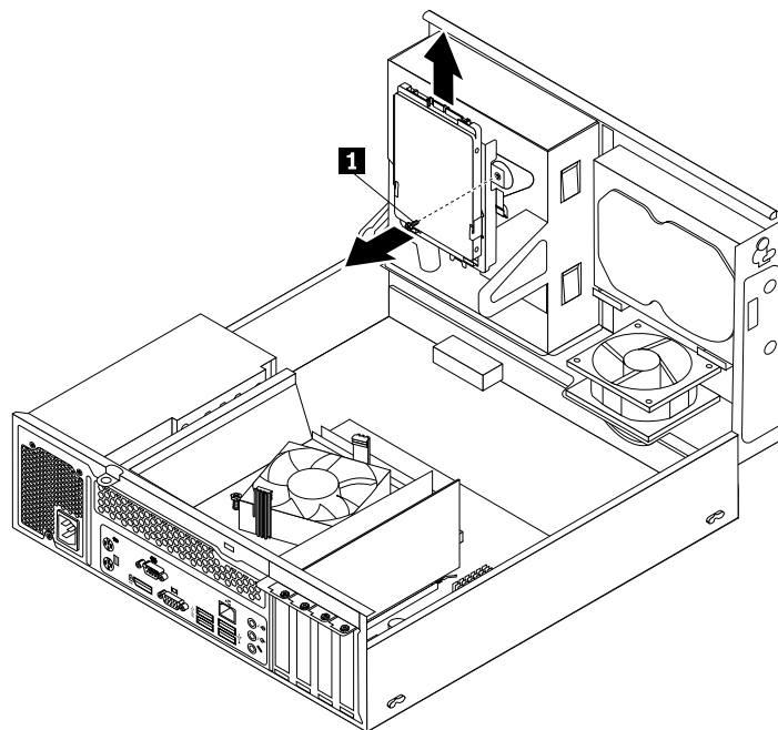
Abbildung 27. Halterung des Solid-State-Laufwerks entfernen
