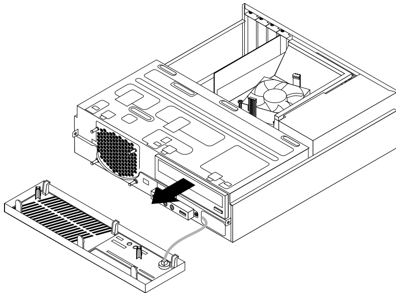
Abbildung 34. Optisches Laufwerk entfernen
