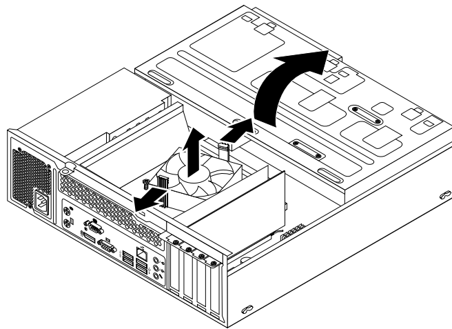
Abbildung 41. Kühlkörperlüftungskanal entfernen
