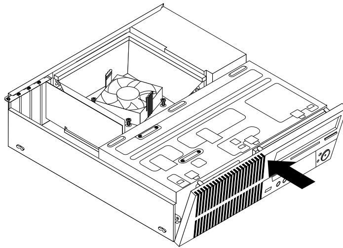
Abbildung 11. Frontblende erneut installieren
