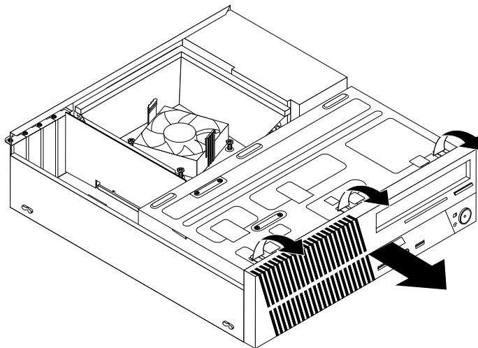
Abbildung 10. Frontblende entfernen
