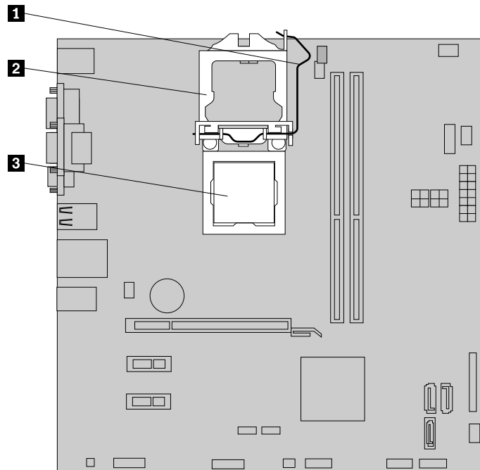
Abbildung 45. Zugriff auf den Mikroprozessor
