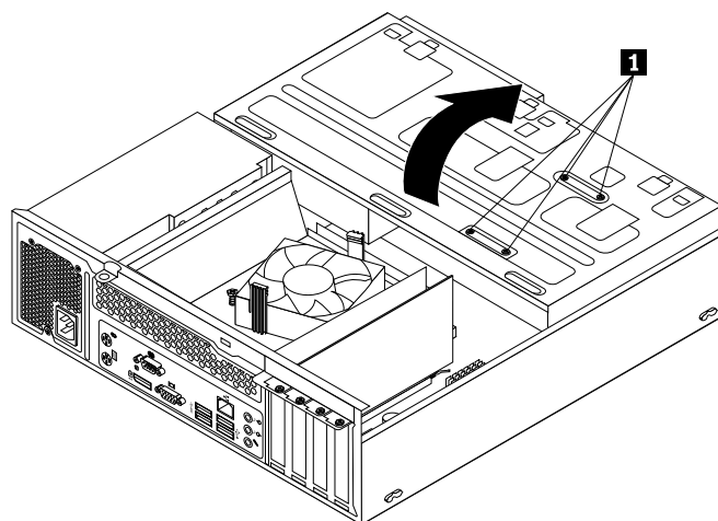
Abbildung 21. Laufwerkposition schwenken
