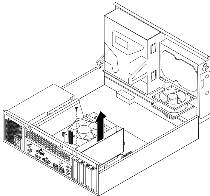
Abbildung 17. PCI-Express-Karte entfernen
