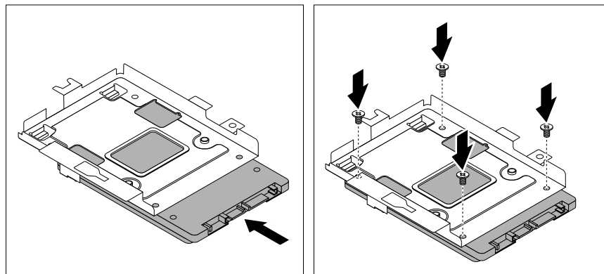
Abbildung 29. Solid-State-Laufwerk in der Halterung einbauen
