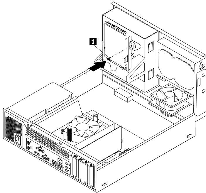
Abbildung 31. Schraube zum Sichern der Halterung am Boden der Position für das optische Laufwerk anbringen
