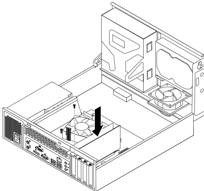
Abbildung 18. PCI-Express-Karte installieren
