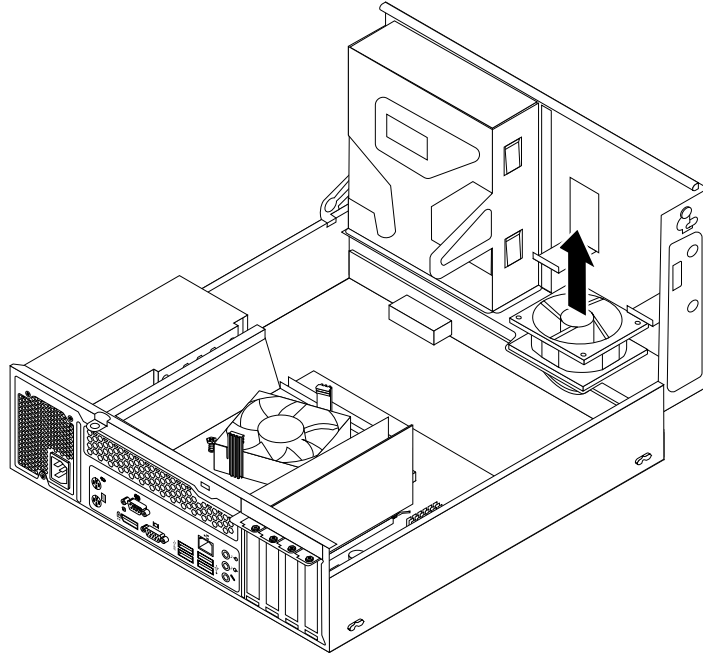
Abbildung 49. Systemlüftungsbaugruppe entfernen
