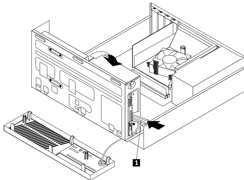
Abbildung 33. Absenken der Laufwerkpositionsbaugruppe
