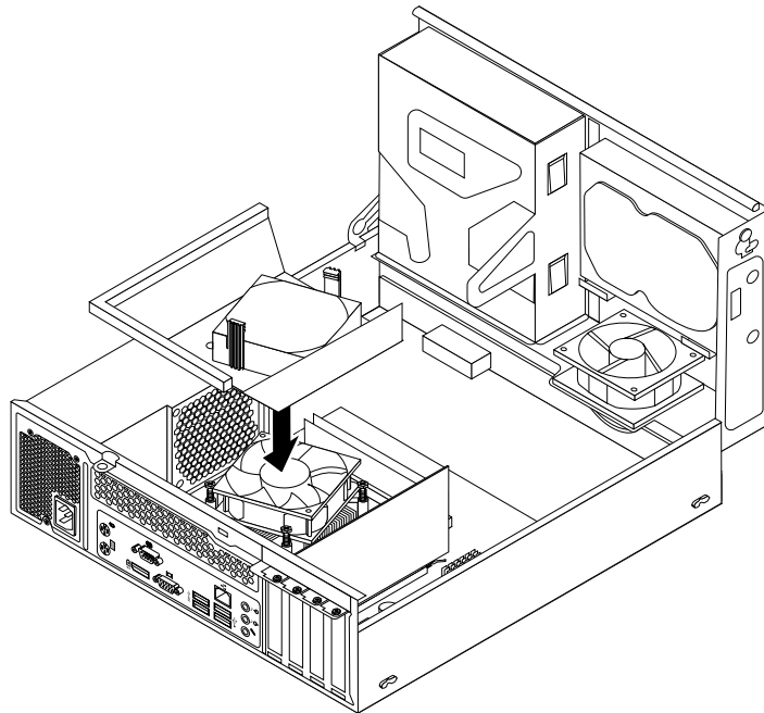
Abbildung 40. Kühlkörperlüftungskanal installieren
