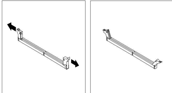
Abbildung 15. Halteklammern öffnen
