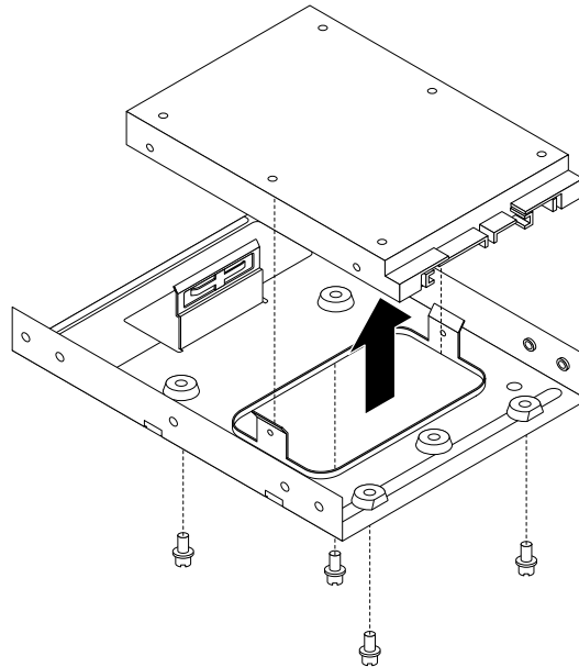
Abbildung 25. Solid-State-Laufwerk aus dem Speicherkonverter entfernen
