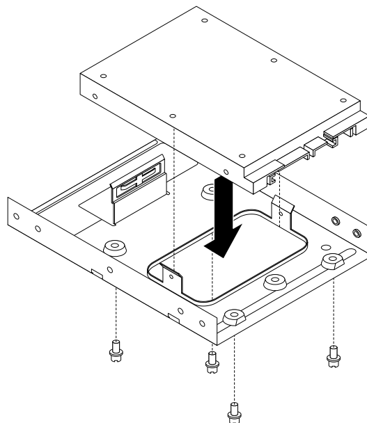
Abbildung 26. Solid-State-Laufwerk im Speicherkonverter installieren
