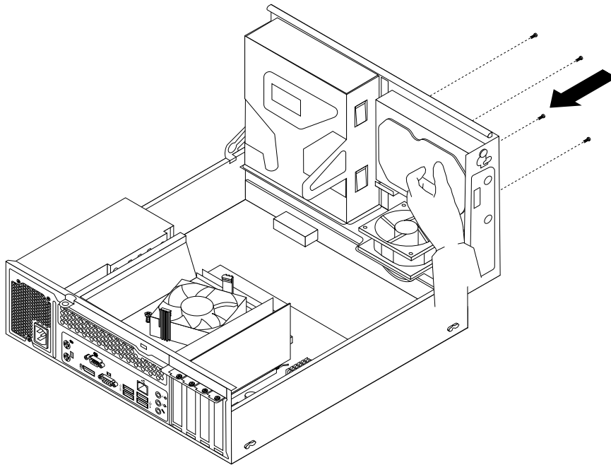
Abbildung 24. Festplattenlaufwerk installieren
