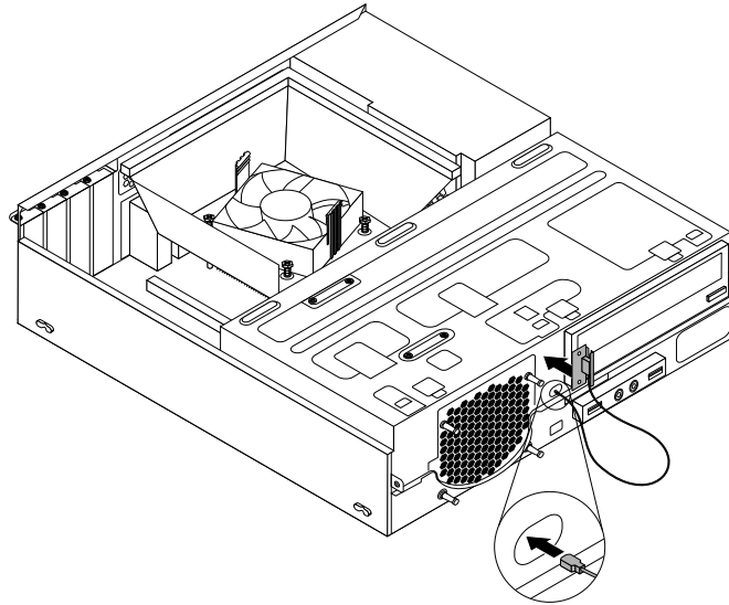
Abbildung 62. Vordere WiFi-Antenne anbringen
