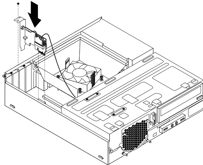
Abbildung 58. WiFi-Adapterkarte installieren
